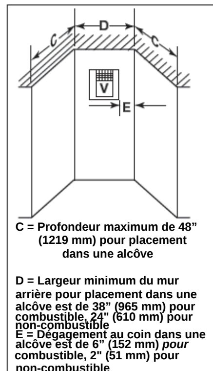
Placement dans une alcôve
