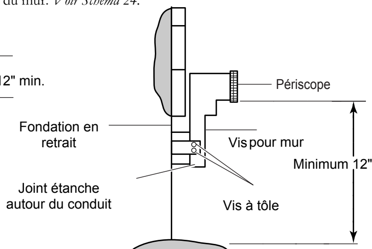
Schéma 24 – Installation du périscopie, fondation en retrait
