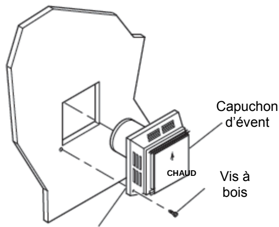
Appliquer du mastic sur les quatre côtés Schéma 14 – Installation du capuchon d'évent horizontal
