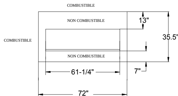
INSTALLATION ENCASTRÉE
