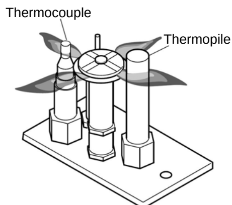
Figure 25 – Avant de démonter l'appareil, vérifier la flamme de la veilleuse. La flamme doit toucher le thermocouple et la thermopile.
