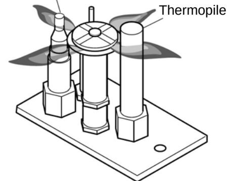
Figure 24 – Apparence normale de la flamme de la veilleuse
