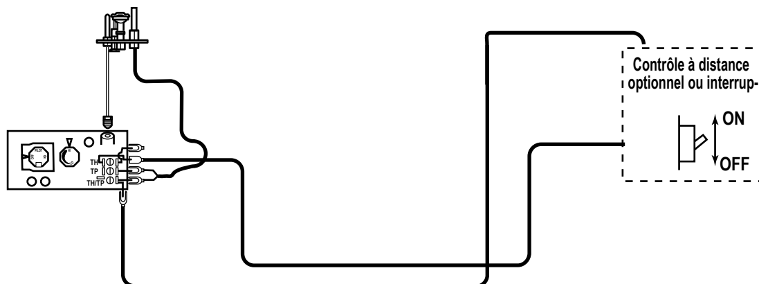
Schéma 35 - Diagramme de branchement pour interrupteur mural.
