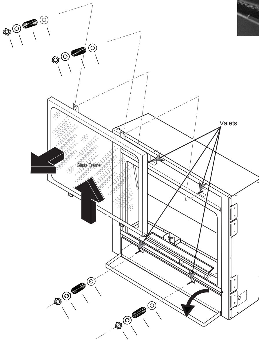
Schéma 36 - Retrait du cadre vitré
