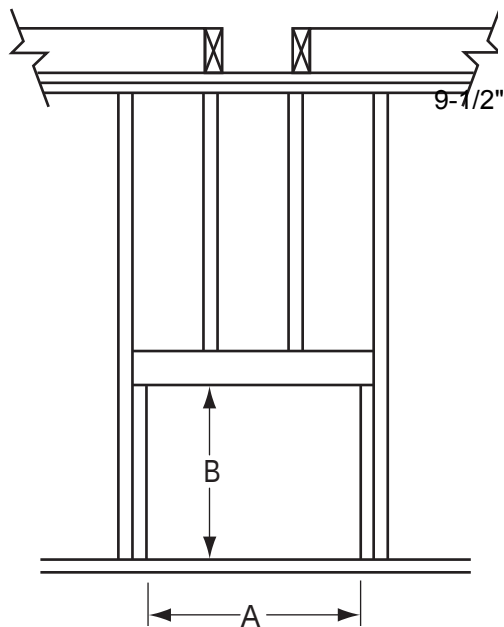
Emplacement des poutres
