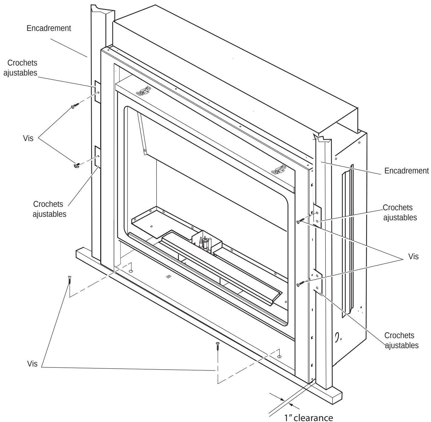
Schéma 5 – Ancrer le foyer au mur et aux crampons du cadre de l'encadrement
