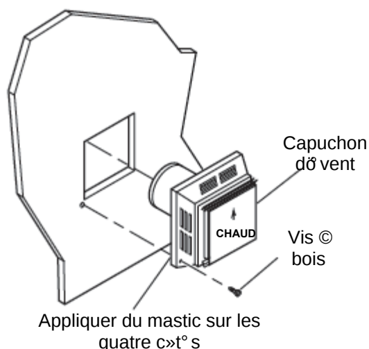
Schéma 14 – Installation du capuchon d'évent horizontal
