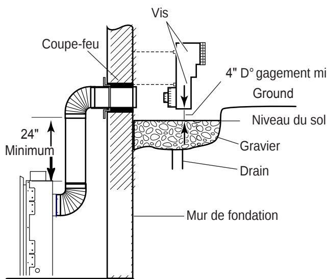
Schéma 23 - Installation souterraine
