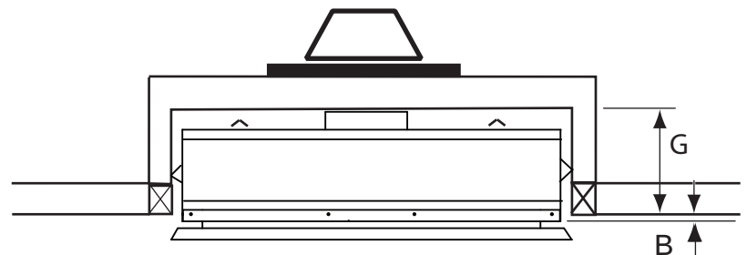
Installation encavée
