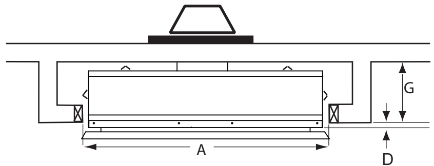
Installation intérieure
